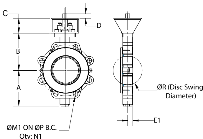
LUG STYLE BODY
